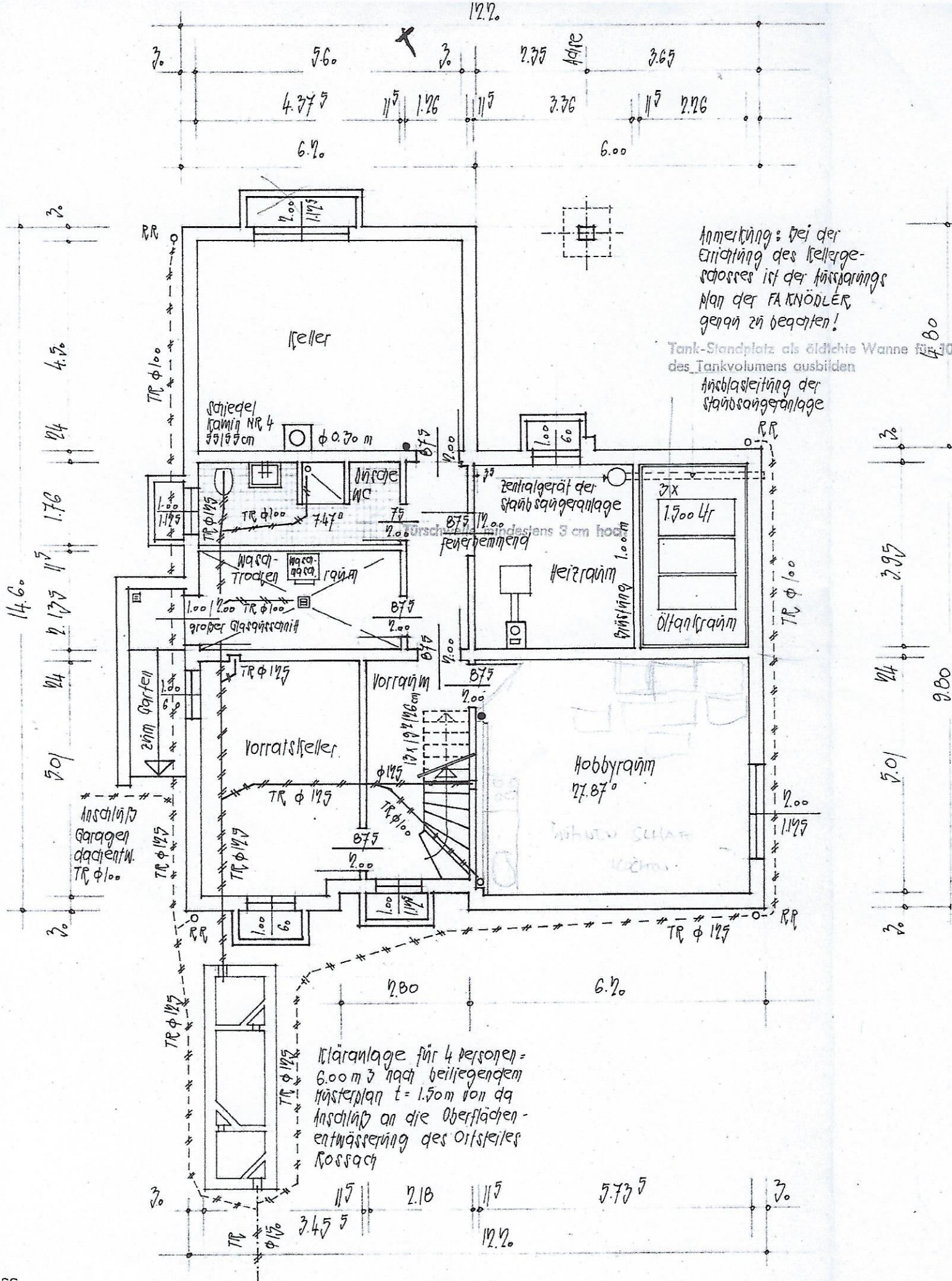
GRUNDRISS KELLERGESCHOSS DARSTELLUNG DER GRUNDSTÜCKSENTWÄSSERUNG
