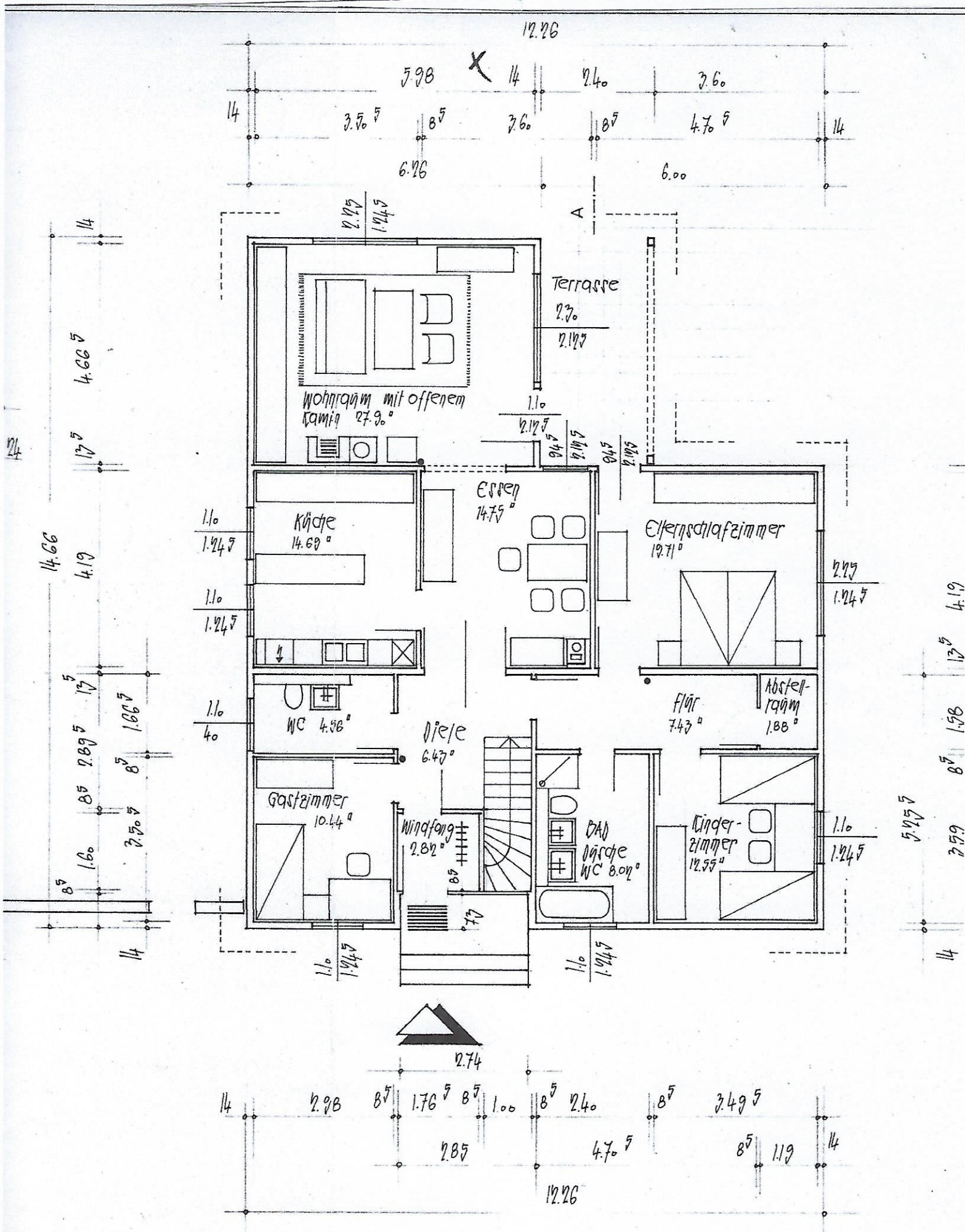
GRUNDRISS ERDGESCHOSS UND DOPPELGARAGE DARSTELLUNG DER GRUNDSTÜCKSGRENZE
