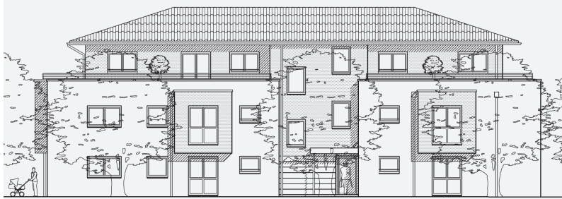
Nord-Westansicht (Eingangsseite) Haus 1
