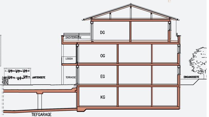
Systemschnitt Haus 1 + 2 (Abb. Haus 2)
