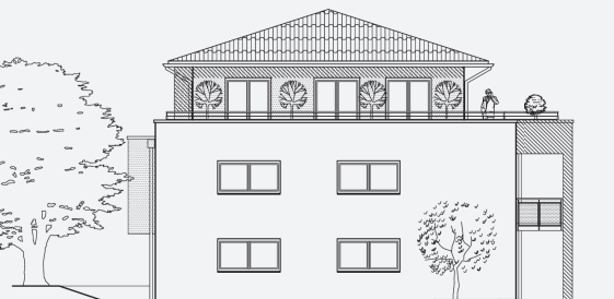
Süd-Westansicht Haus 1
